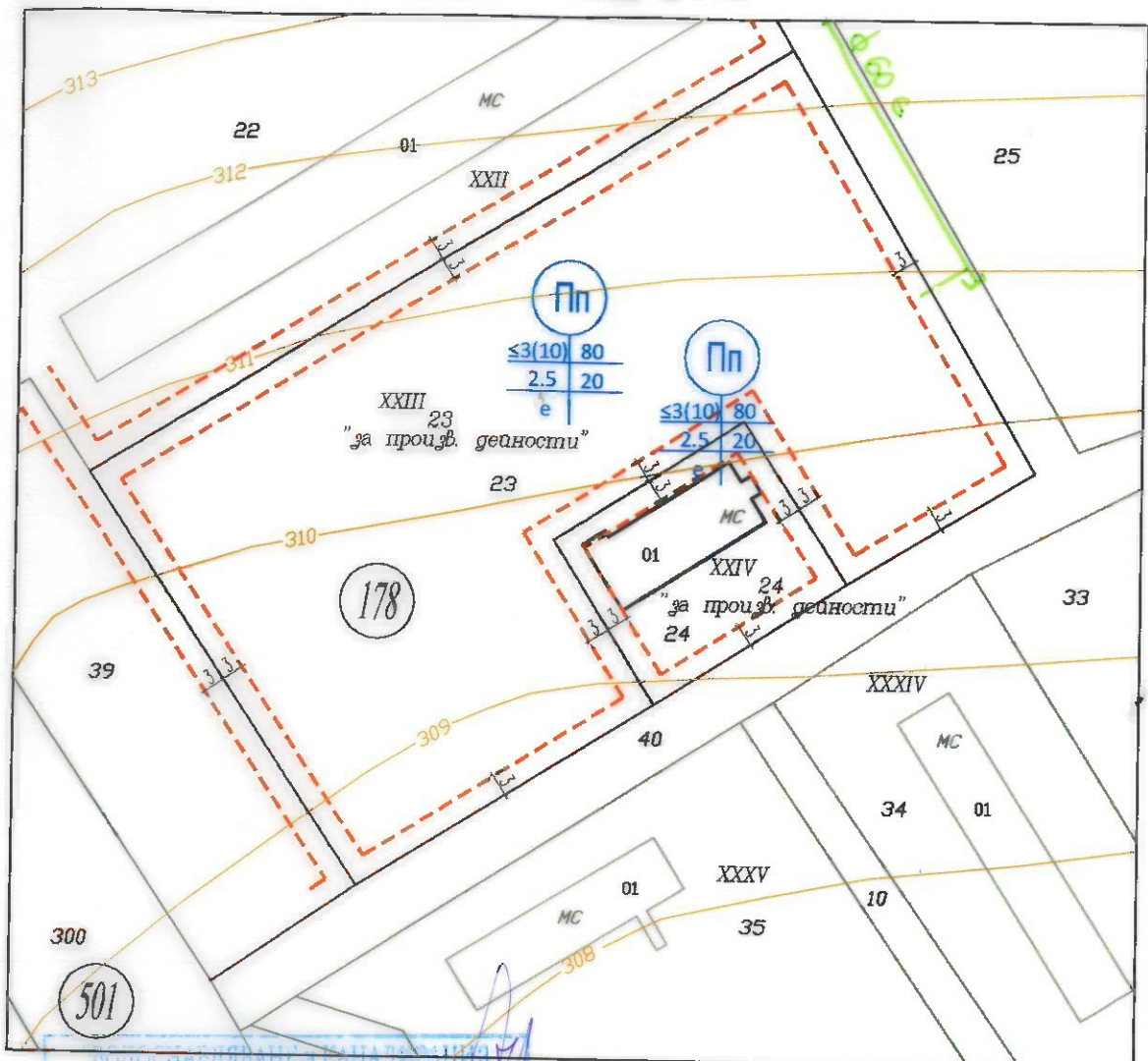
ПЛАН за ЗАСТРОЯВАНЕ - М 1:1000
